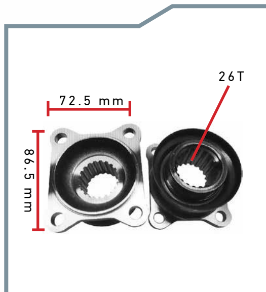
FLANGE
