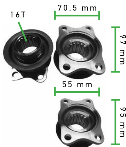
FLANGE
